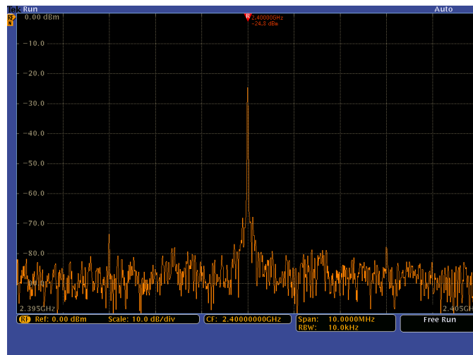
Отображение частотной области на экране MDO4000B.
